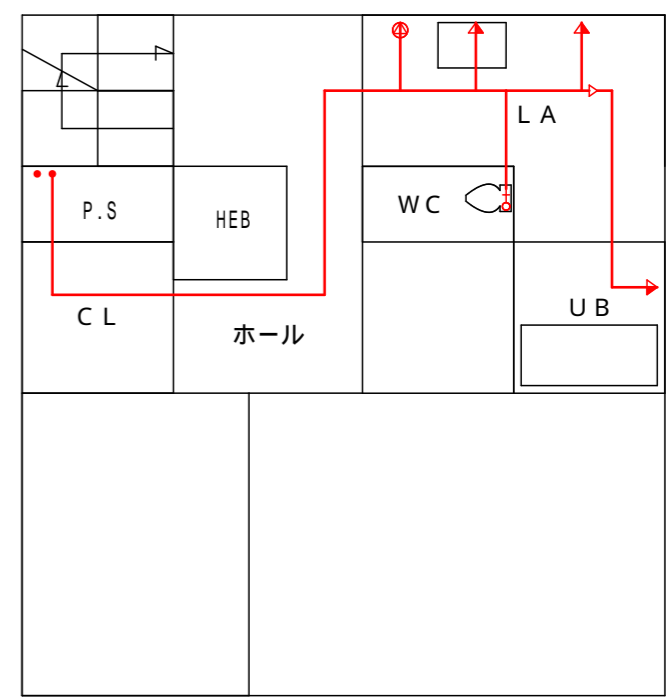
2 F 平面図
