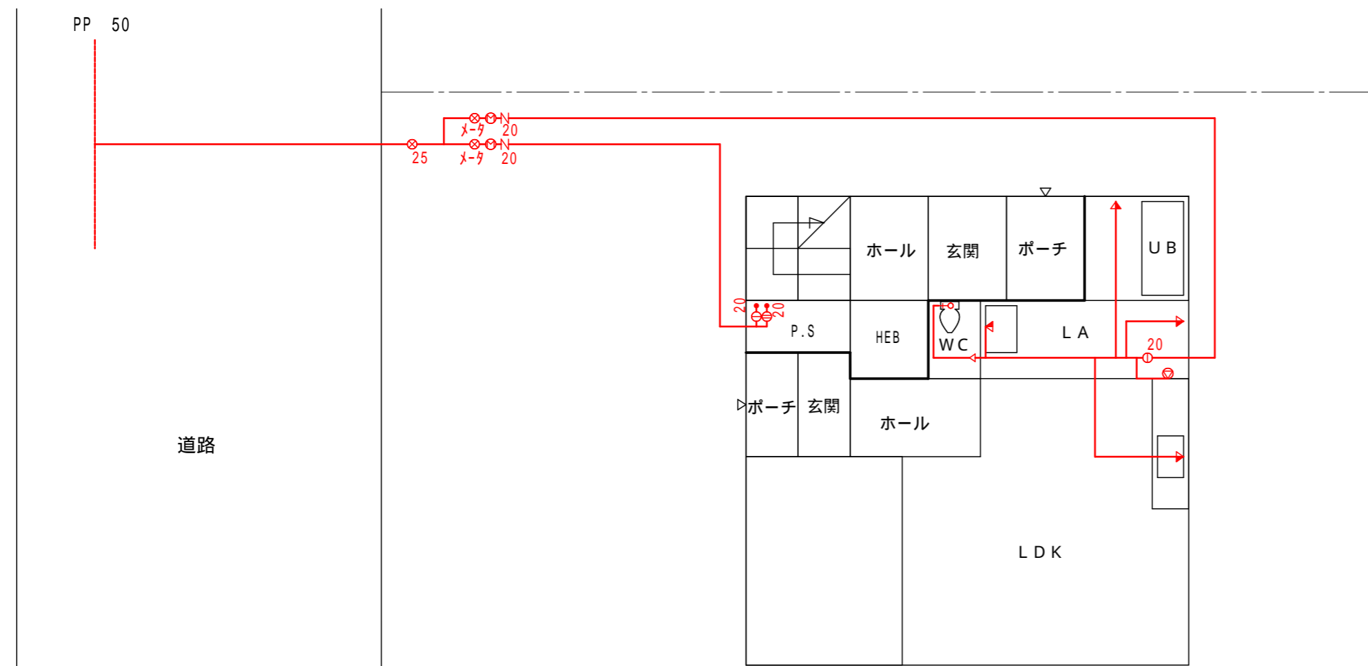
1 F 平面図
